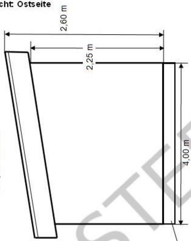
Beispiel Pultdach
